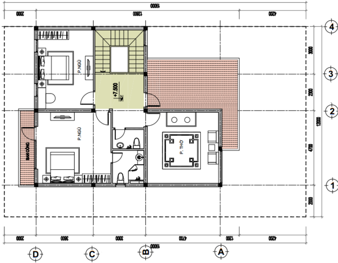
MẶT BẰNG TẦNG 3
